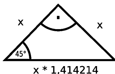
Abbildung 6: Rechtwinkliges Dreieck
